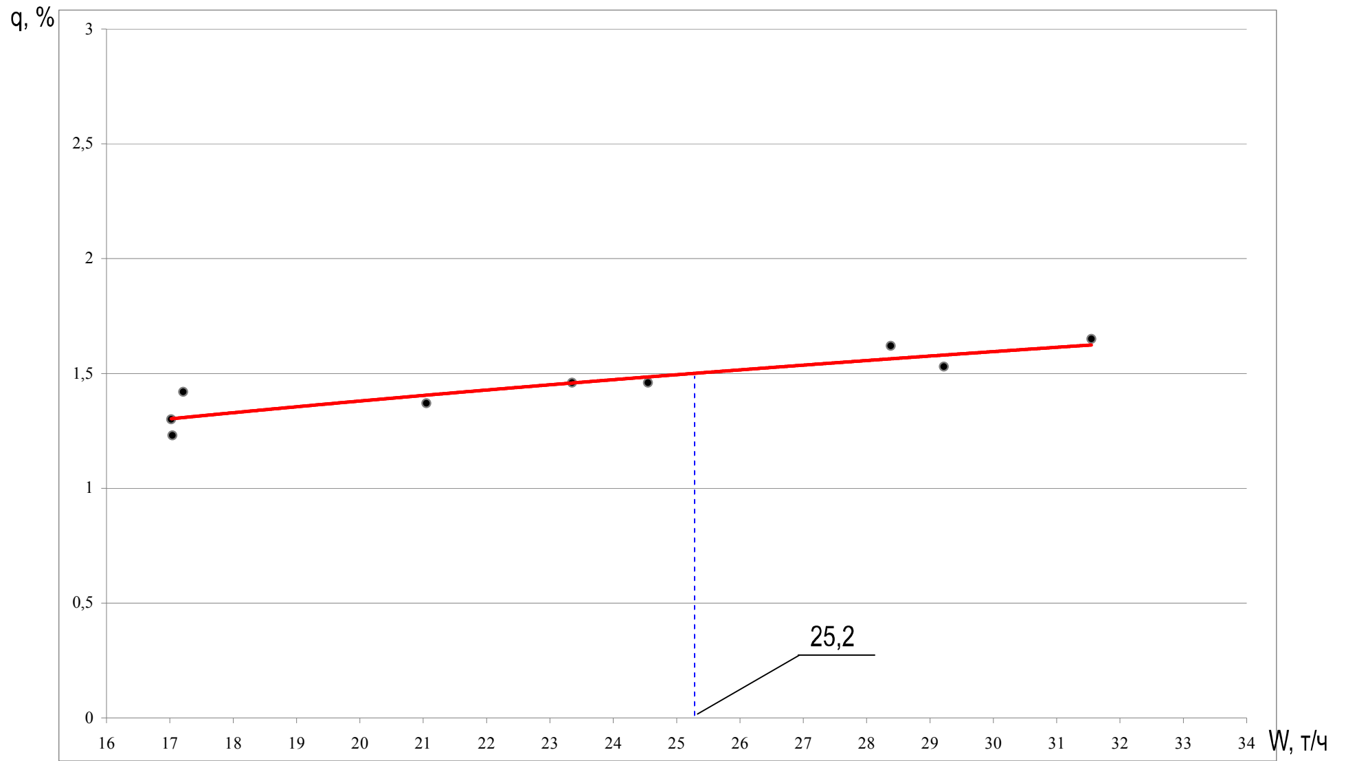
График зависимости потерь зерна молотилкой комбайна от производительности
