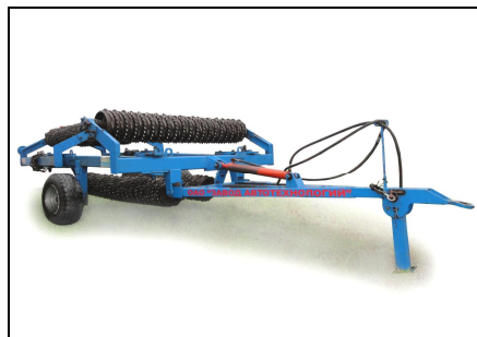
Каток кольчато-зубчатый ККЗ-9,2Н, вид спереди справа
