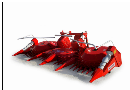
Приспособление для уборки кукурузы на силос Kemper 445, вид спереди слева
