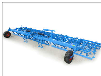
Культиватор Korund 8/900 К (вид спереди слева)
