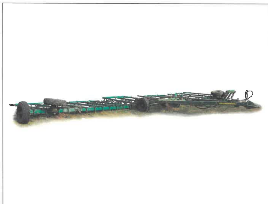
Рисунок 1 – Борона широкозахватная гидрофицированная БШГ -15-К1 "Пустельга", вид спереди справа
