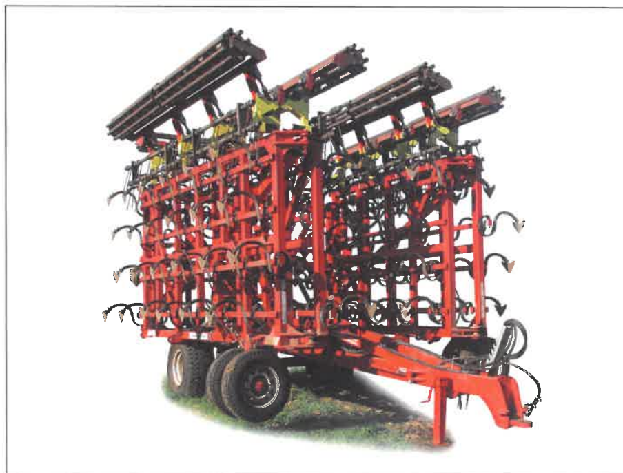
Рисунок 1 – Средний предпосевной культиватор "Tillermaster-18000", в транспортном положении
