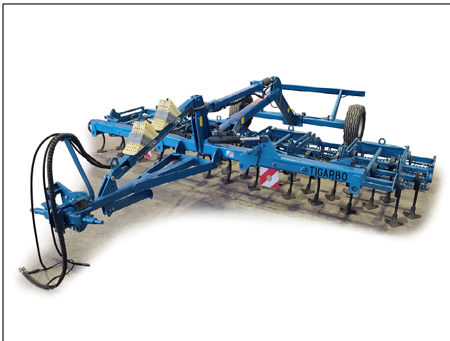
Рисунок 1 – Культиватор предпосевной торговой марки "TIGARBO" модель КПП-6, в положении хранения
