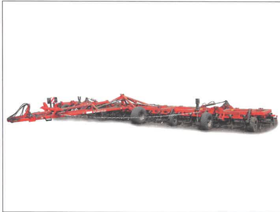
Рисунок 1 – Культиватор сплошной, серии КС(У), модели КС-14(УС)-03.00 EURO, вид спереди слева
