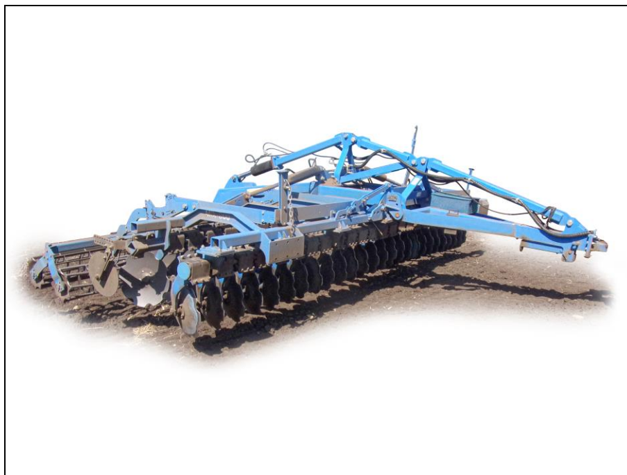
Рисунок 1 – Борона дисковая МІХ-800, вид спереди справа
